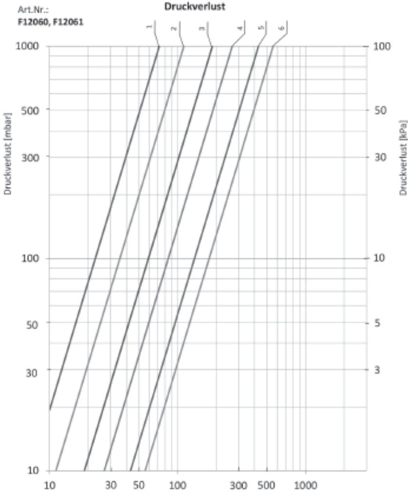
Bild 2: Druckverlustdiagramm
